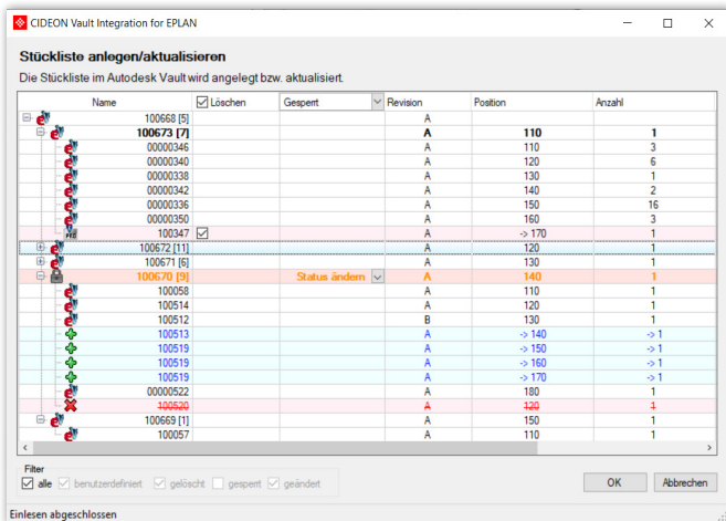
Stücklistenanlage/Aktualisierung bei neuen, geänderten oder gesperrten Positionen
